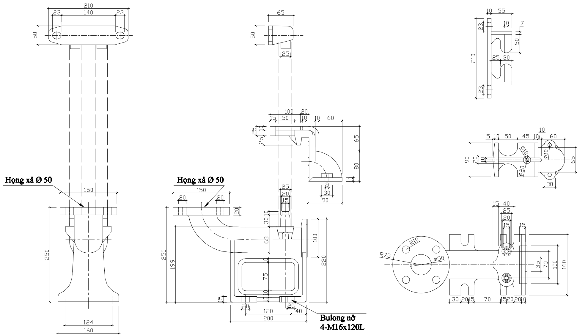
Kích thước khớp nối nhanh TOS5-50
